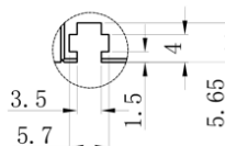
视图A (两边对称) 2:1
