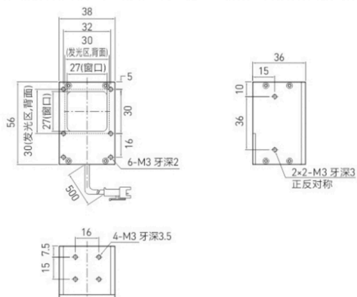
LS-COS30-ZT
