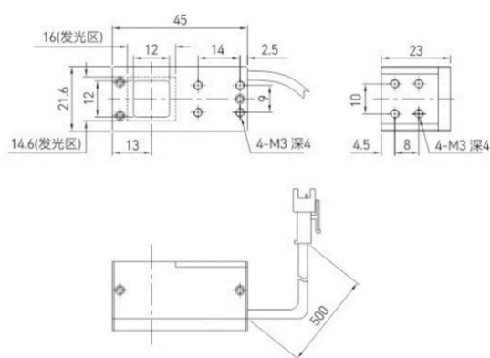
LS-COS30-ZT
