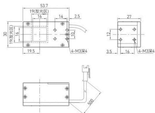
LS-COS40-ZT
