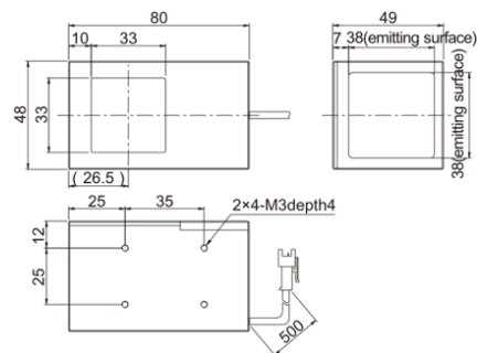
6.LS-2COXR100
