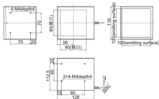
6.LS-2COXR100
