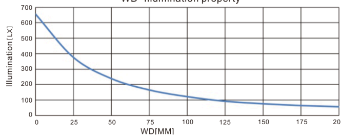
WD-Illumination property
