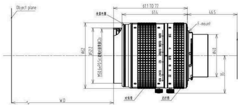
LS-MF5015A
