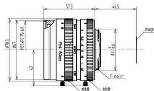
LS-MF6016A
