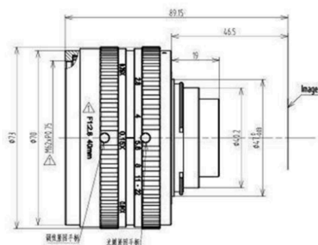
LS-MF4010A
