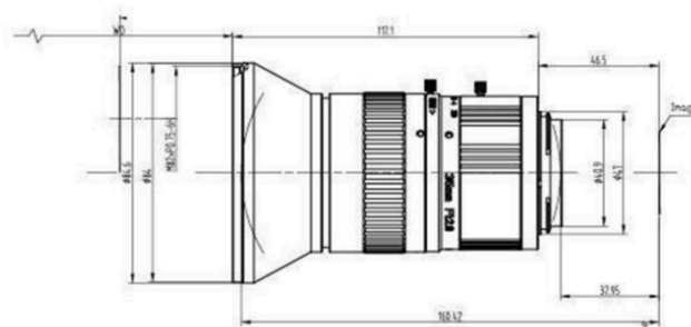
LS-MF3515A
