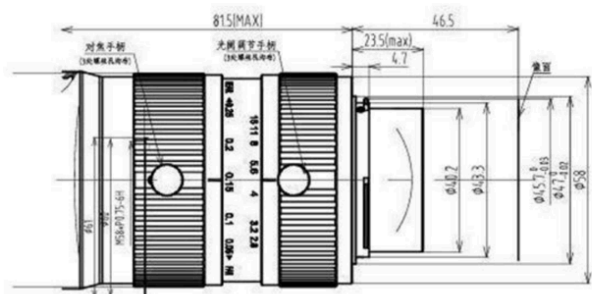
LS-MF3502A
