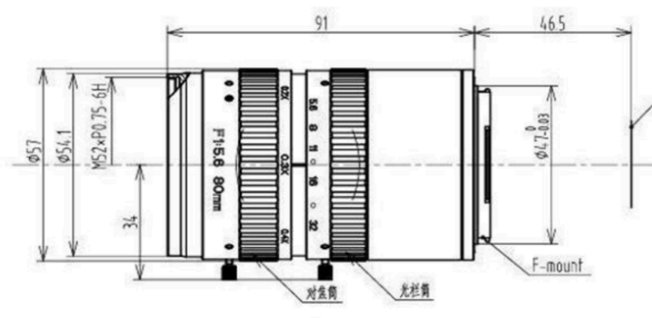
LS-MF8003A
