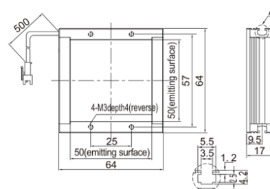
6.LS-2FT5050
